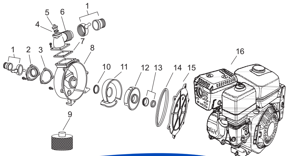
DIAGRAMA DE PARTES
